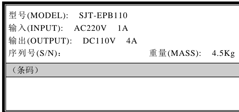
图 1.2 铭牌说明示意图
