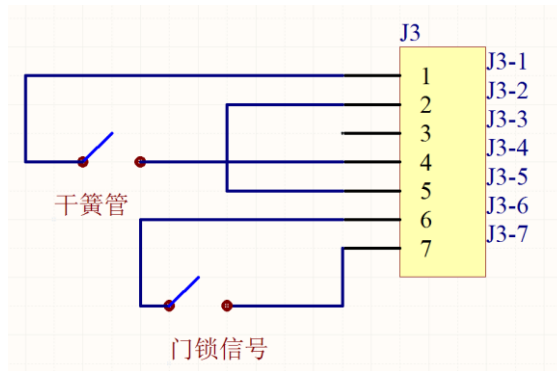
图 2.4 门区信号接入方式 2
