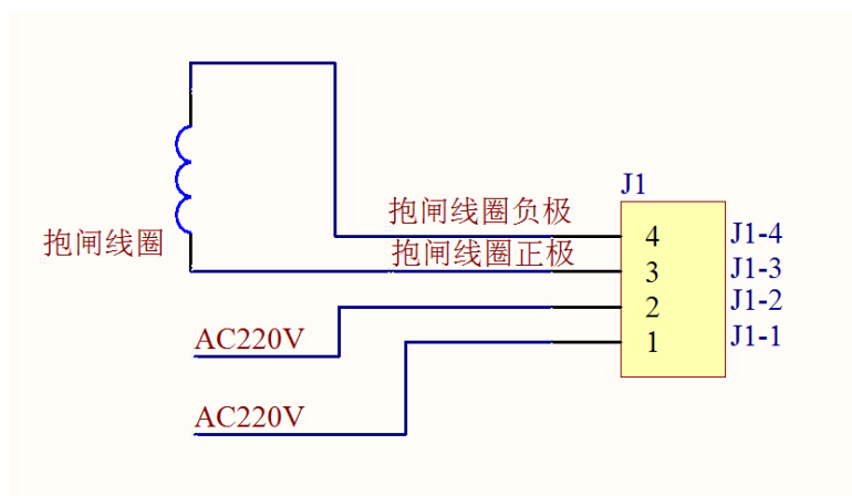
图 2.1 输入输出接线
