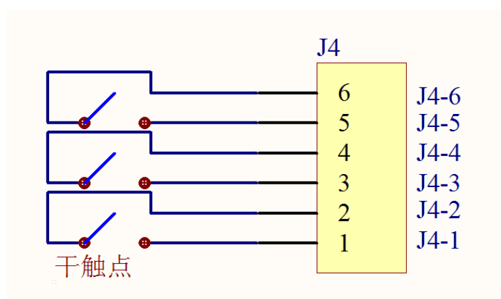
图 2.7 按键信号接入方法
