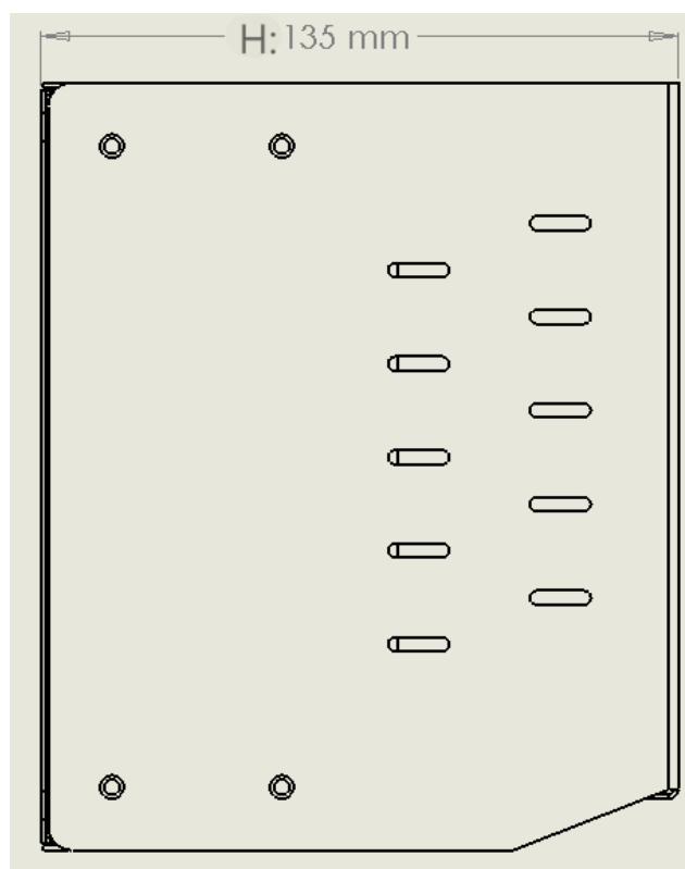
图 1.4 侧面外形尺寸
