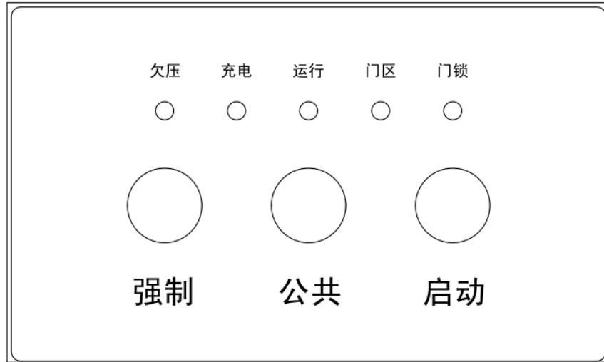
图 3.1 操作面板外观示意图
