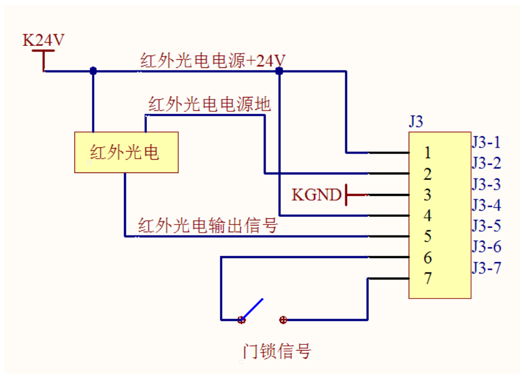
图 2.6 门区信号接入方法 4
