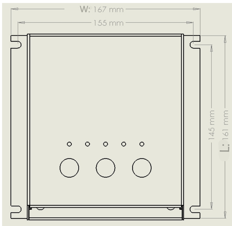
图 1.3 正面外形尺寸
