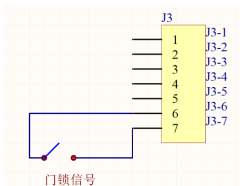
图 2.2 门锁信号接入方法
