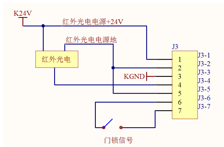
图 2.5 门区信号接入方式 3
