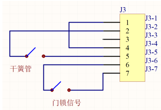
图 2.3 门区信号接入方式 1
